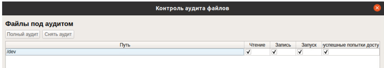
Рисунок 90. Вкладка «Аудит файлов»
