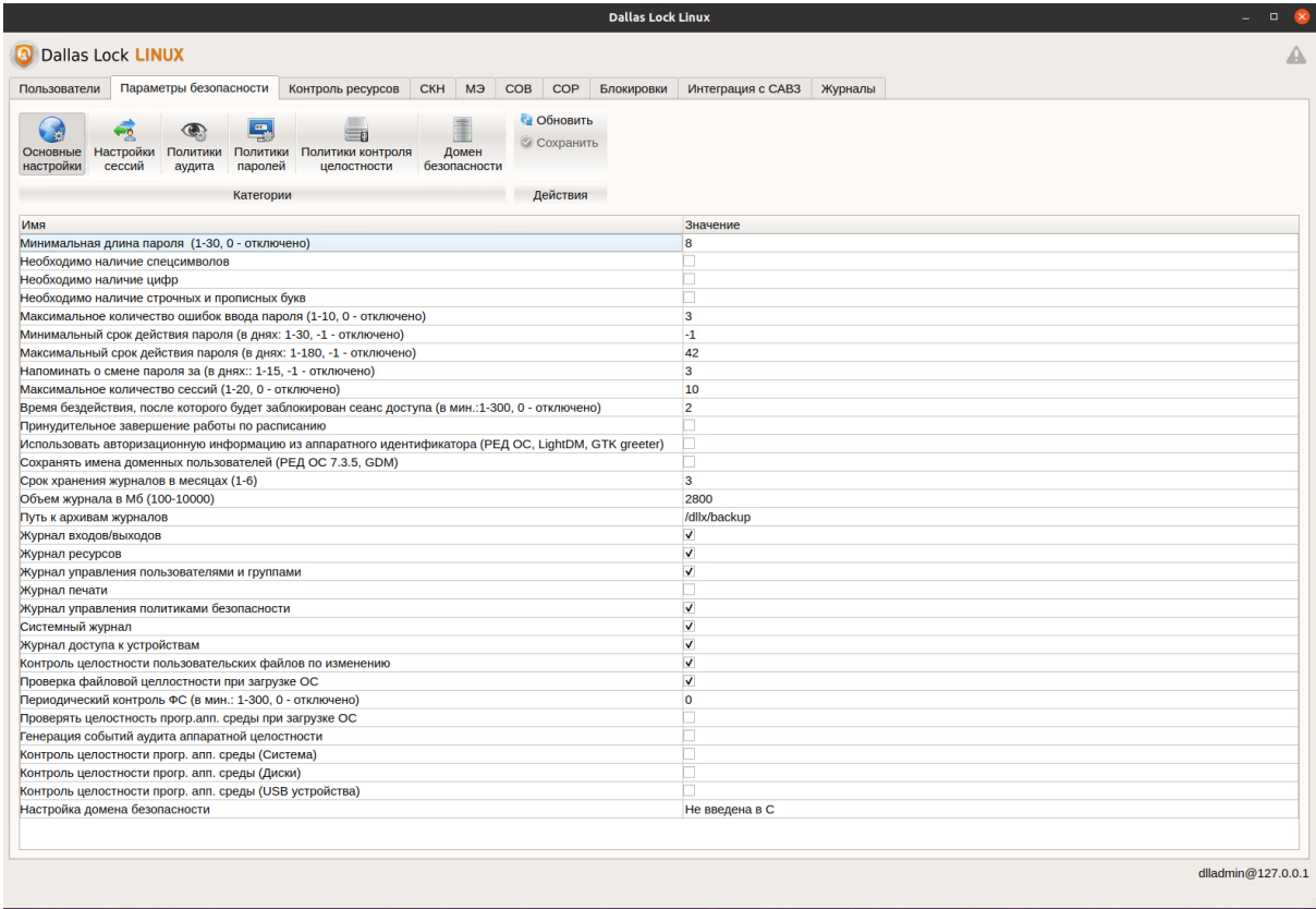
Рисунок 51. Вкладка «Параметры безопасности» с модулем НСД
