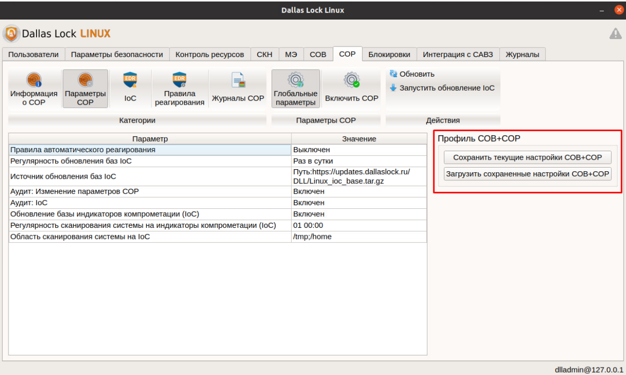
Рисунок 207. Управление профилем COB+COB
