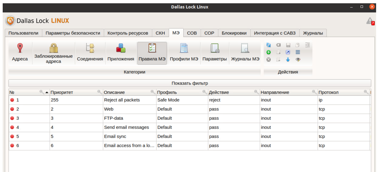
Рисунок 110. Список настроенных правил МЭ
