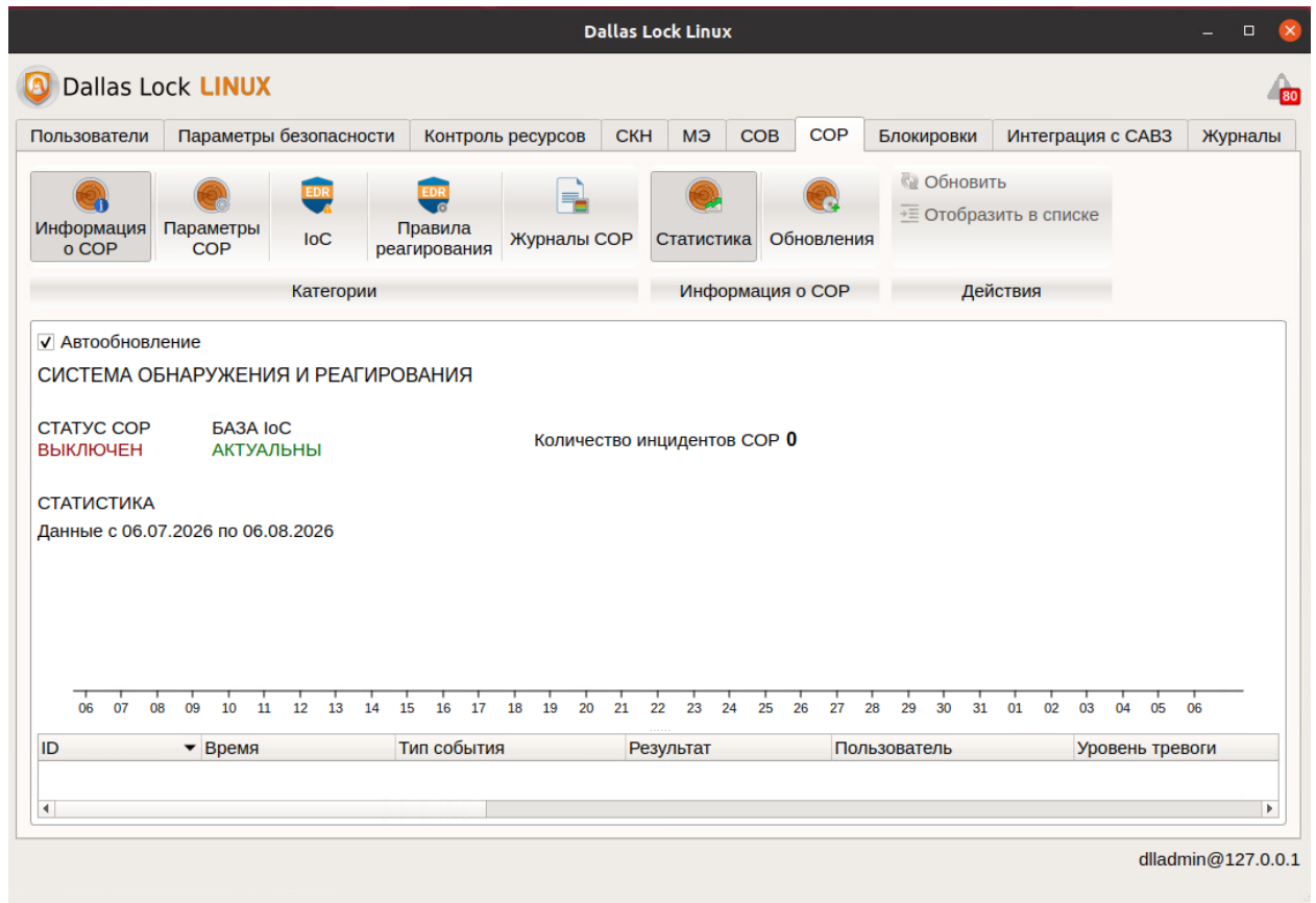
Рисунок 193. Вкладка «СОР» в графической оболочке администрирования
